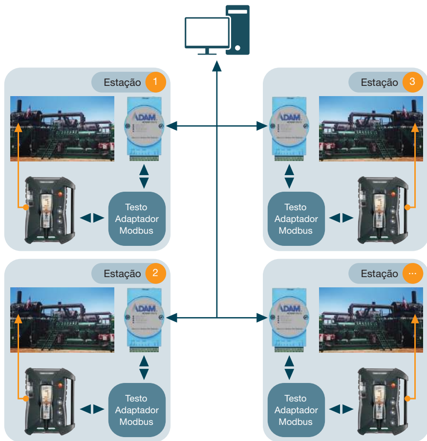
Figura 61 Exemplo de aplicação do adaptador Modbus
