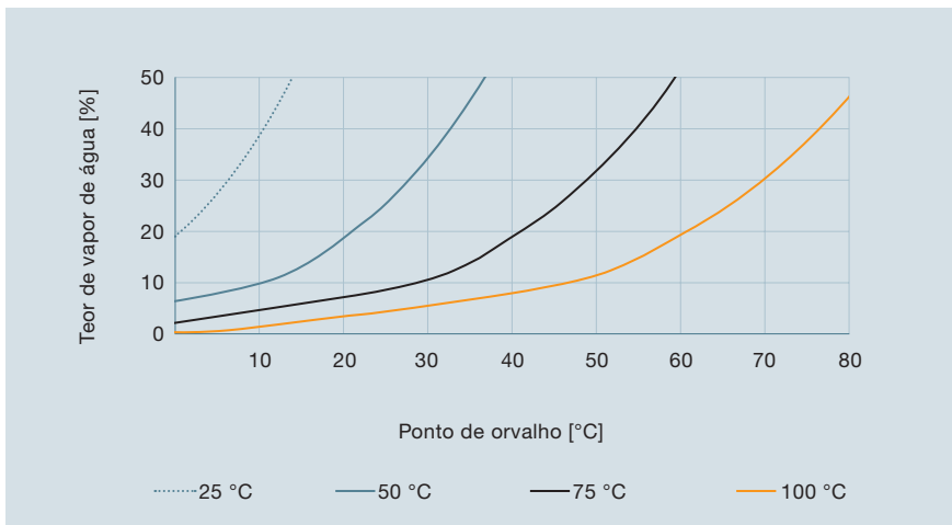
Figura 5 Teor de vapor de água em função do ponto de orvalho em diferentes temperaturas ambientes (pressão atmosférica 1013 mbar).
