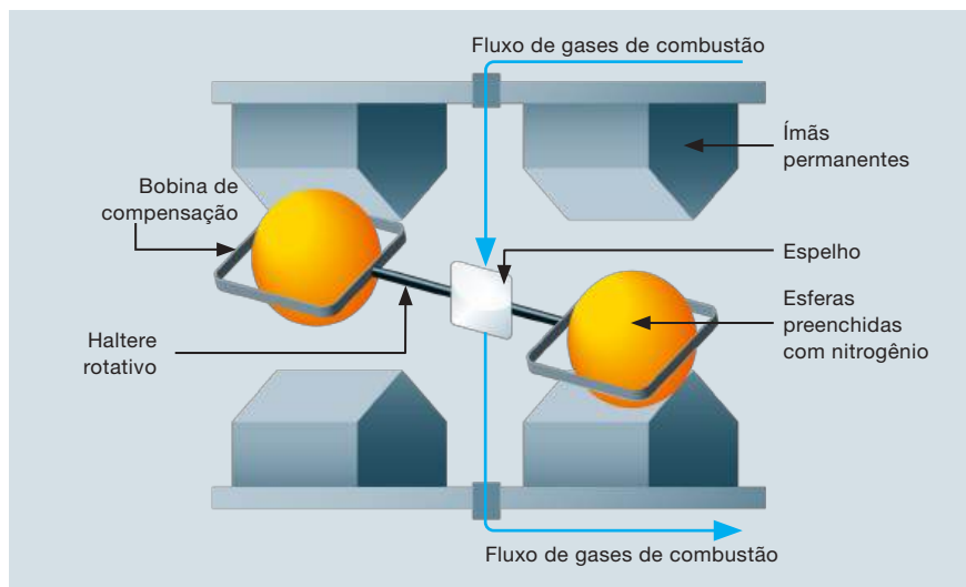
Figura 20 Sensor paramagnético
