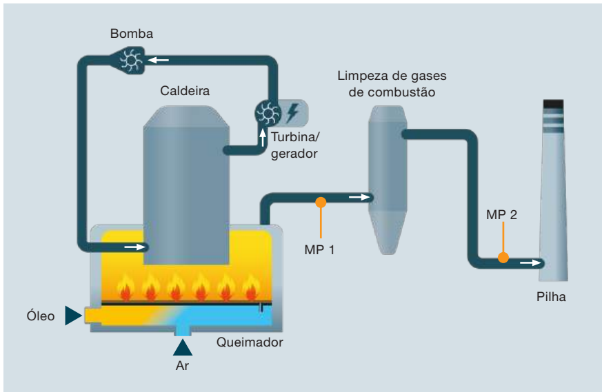
Figura 30 Fluxograma de processo para uma instalação a óleo com pontos de medição
