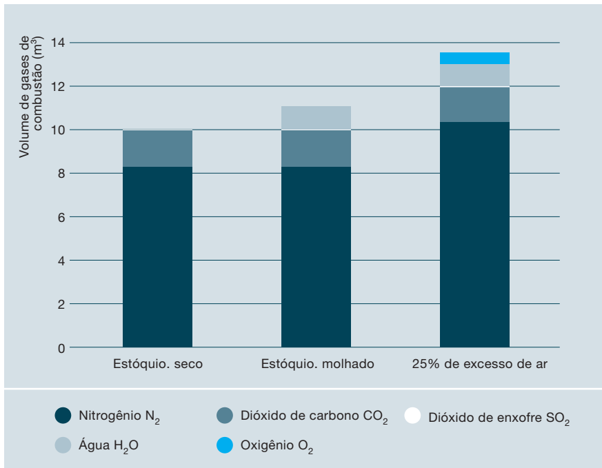
Figura 4 Efeito diluidor do teor de umidade e do excesso de ar
