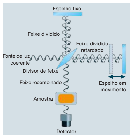
Figura 24 Espectroscopia de infravermelho com transformada de Fourier (FTIR)
