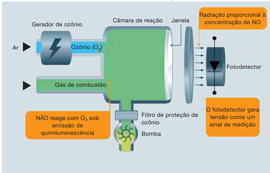
Figura 19 Método CLD
