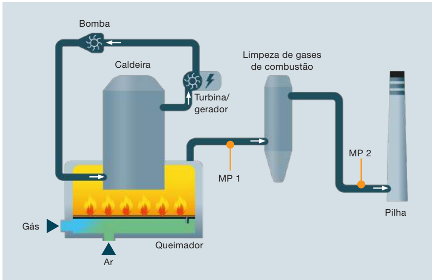
Figura 28 Fluxograma de processo para uma instalação a gás com pontos de medição
