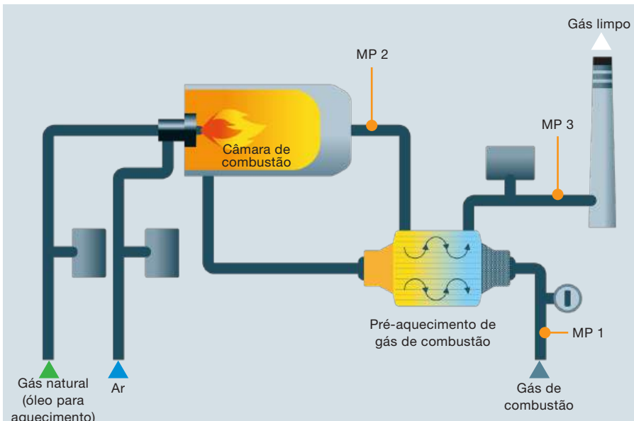
Figura 37 Fluxograma do processo para uma instalação de pós-combustão térmica com pontos de medição
