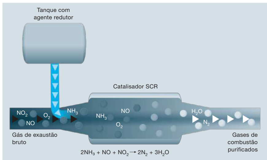
Figura 12 Representação esquemática do processo SCR
