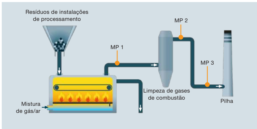
Figura 52 Fluxograma de processo para uma planta de incineração de resíduos com pontos de medição
