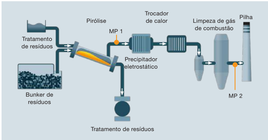
Figura 36 Fluxograma de processo para uma instalação de pirólise de resíduos com pontos de medição
