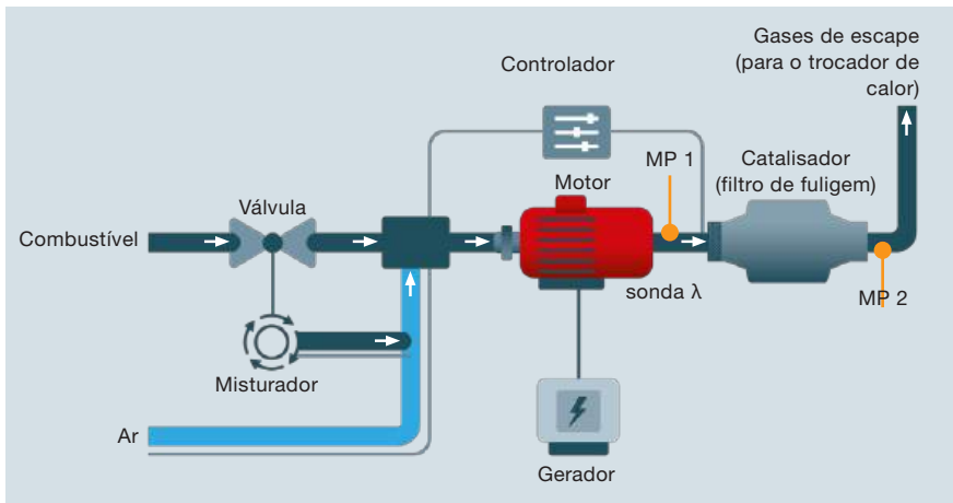
Figura 32 Fluxograma de processo para o motor de uma usina de cogeração (CHP)
