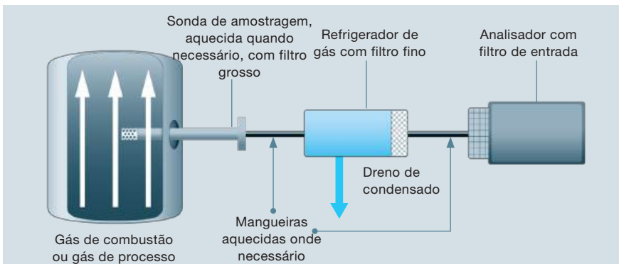
Figura 13 Extração e condicionamento do gás de amostra (esquemático)
