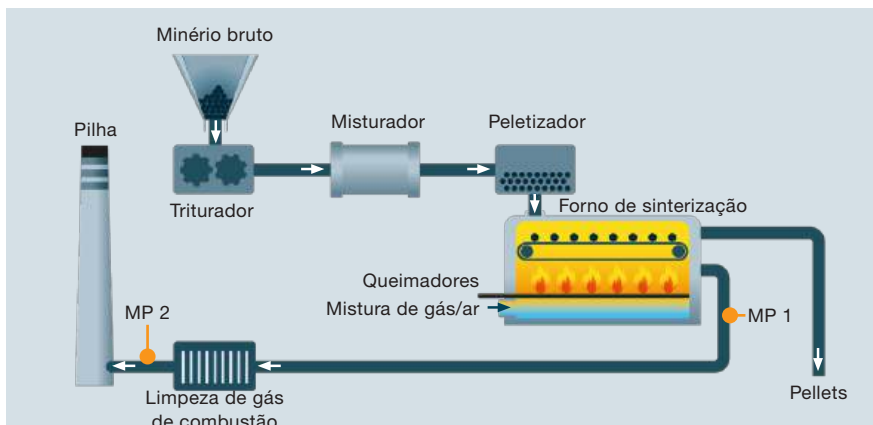
Figura 43 Fluxograma do processo de produção de pelotas (sinterização) com pontos de medição
