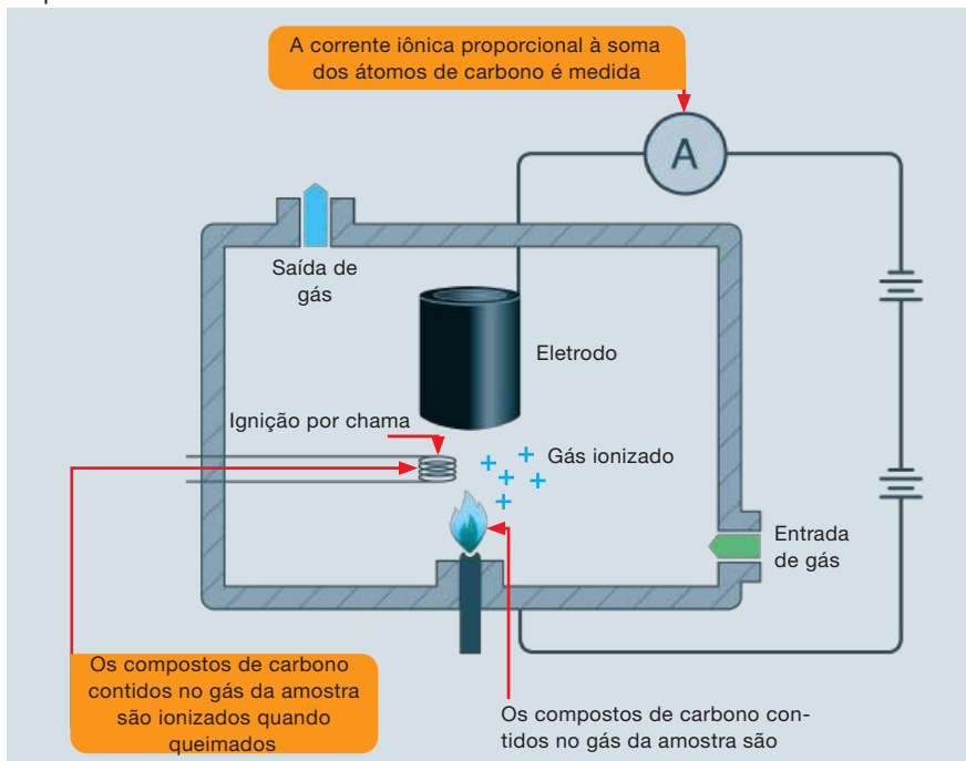
Figura 23 Detector de ionização de chama
