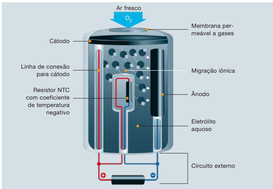
Figura 16 Sensor de oxigênio (esquemático)
