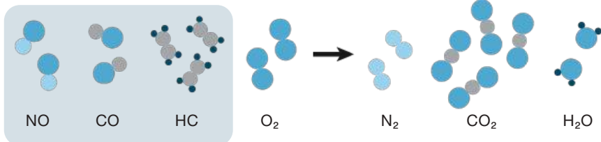
Figura 11 Conversão de poluentes em um catalisador de três vias
