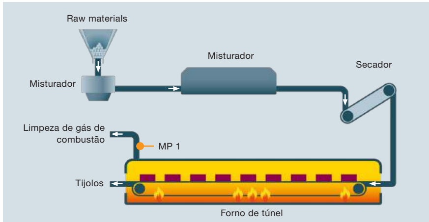
Figura 40 Fluxograma do processo de produção de tijolos com ponto de medição
