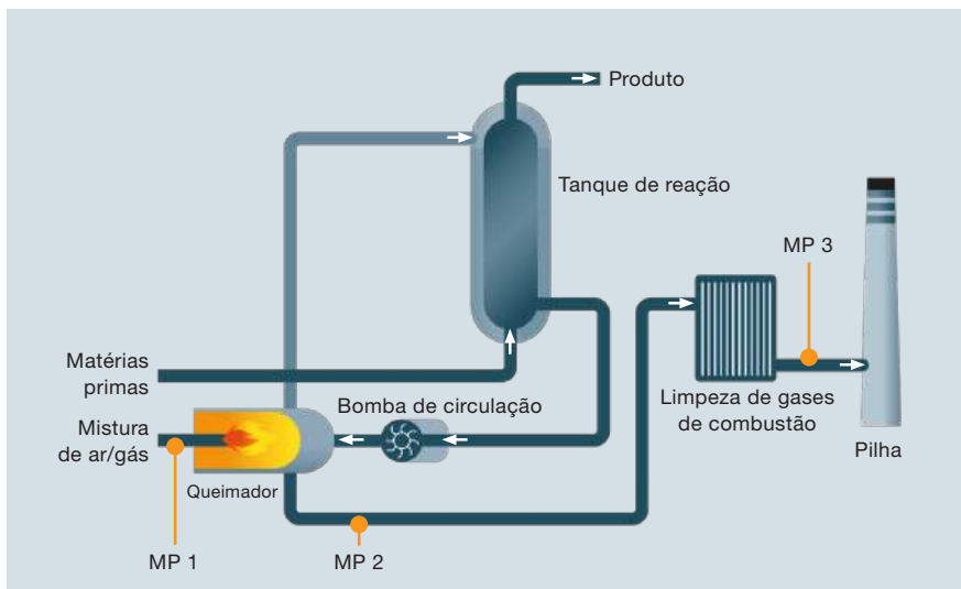
Figura 49 Fluxograma de processo para um aquecedor de processo com pontos de medição
