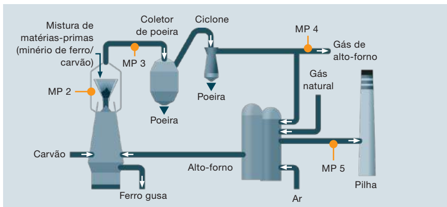
Figura 44 Fluxograma do processo de produção de ferro gusa (w) com pontos de medição
