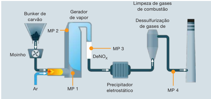
Figura 31 Fluxograma de processo para uma usina elétrica a carvão com pontos de medição
