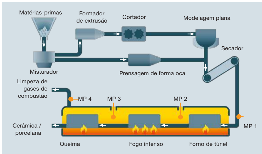
Figura 39 Fluxograma de processo para produção de cerâmica/porcelana com pontos de medição
