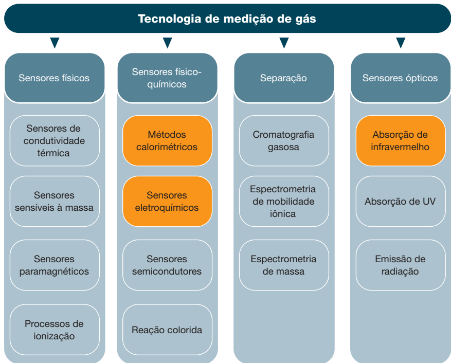
Figura 15 Métodos de tecnologia de medição de gás
