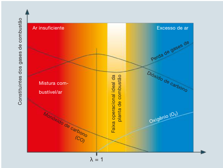
Figura 3 Gráfico de combustão
