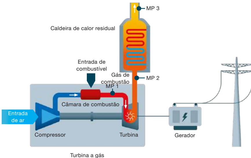
Figura 29 Fluxograma de processo para uma usina de turbina a gás com pontos de medição
