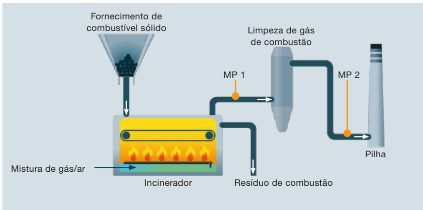
Figura 27 Fluxograma do processo de um sistema alimentado por combustível sólido com pontos de medição
