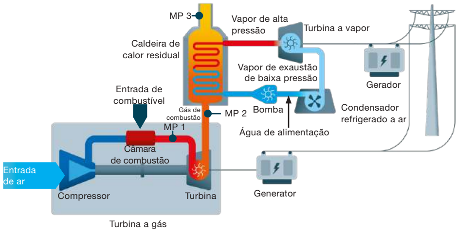
Figura 33 Fluxograma de processo para uma usina de ciclo combinado com pontos de medição
