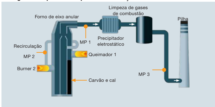
Figura 42 Fluxograma do processo de produção de cal com pontos de medição
