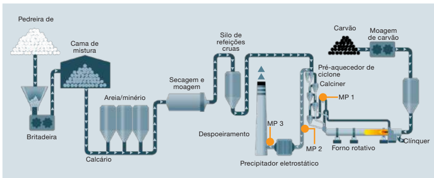
Figura 38 Fluxograma do processo de produção de cimento com pontos de medição
