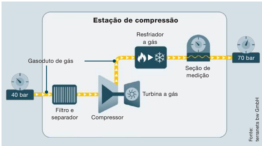
Figura 34 Fluxograma de processo para uma estação de compressão
