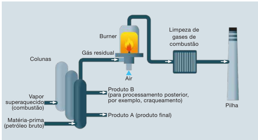
Figura 50 Fluxograma de processo para uma refinaria (sem pontos de medição)
