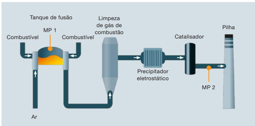
Figura 28: Fluxograma do processo para planta de produção de vidro com pontos de medição
