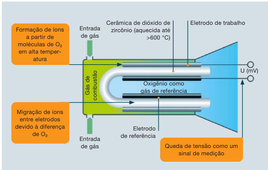
Figura 25 Sensor de óxido de zircônio
