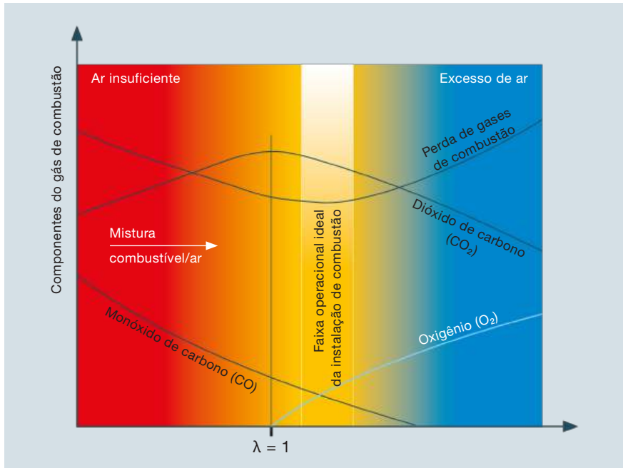
Figura 7 Gráfico de combustão
