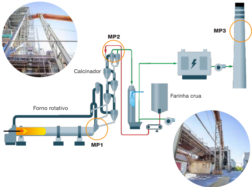
Figura 8 Representação esquemática de uma planta de cimento com pontos de medição (MP) típicos para utilização de analisadores
