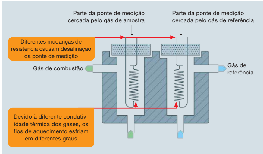
Figura 21 Detector de condutividade térmica
