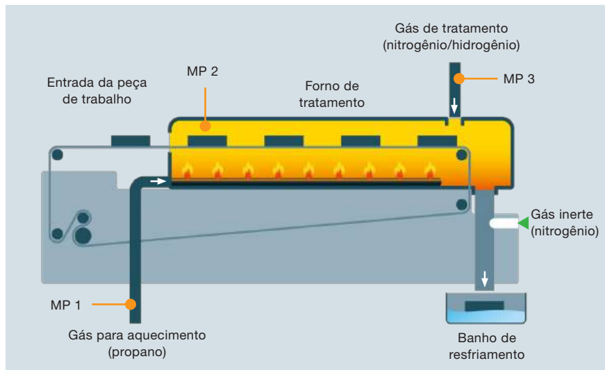
Figura 48 Diagrama de um forno para tratamento de superfície com pontos de medição
