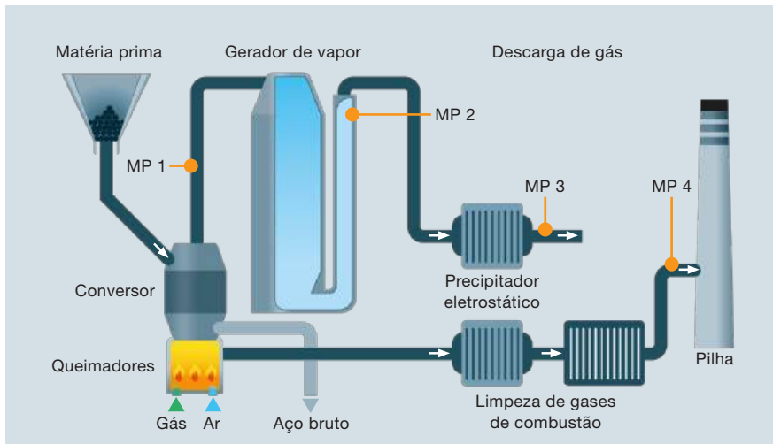
Figura 45 Fluxograma do processo de produção de aço bruto com pontos de medição
