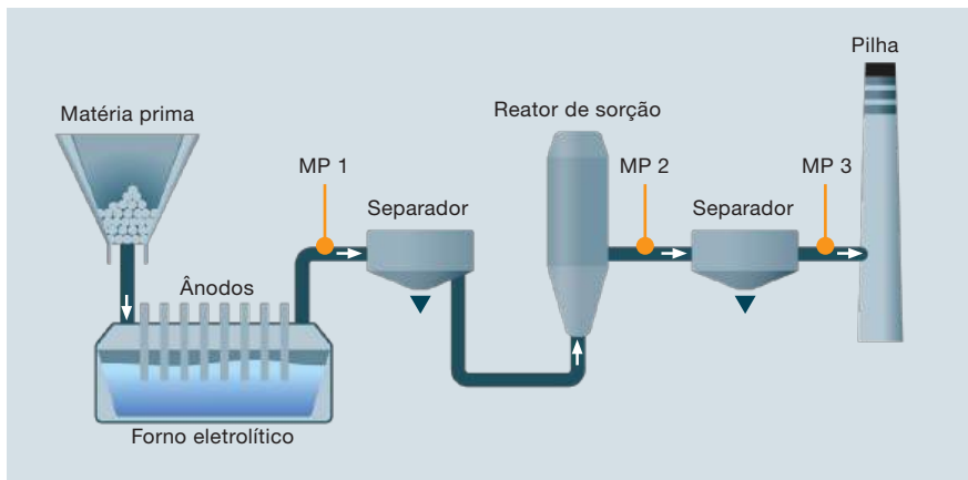
Figura 47 Fluxograma do processo de produção de alumínio com pontos de medição
