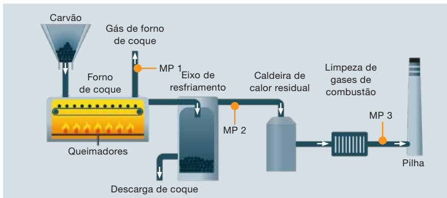
Figura 46 Fluxograma de processo para uma coqueria com pontos de medição
