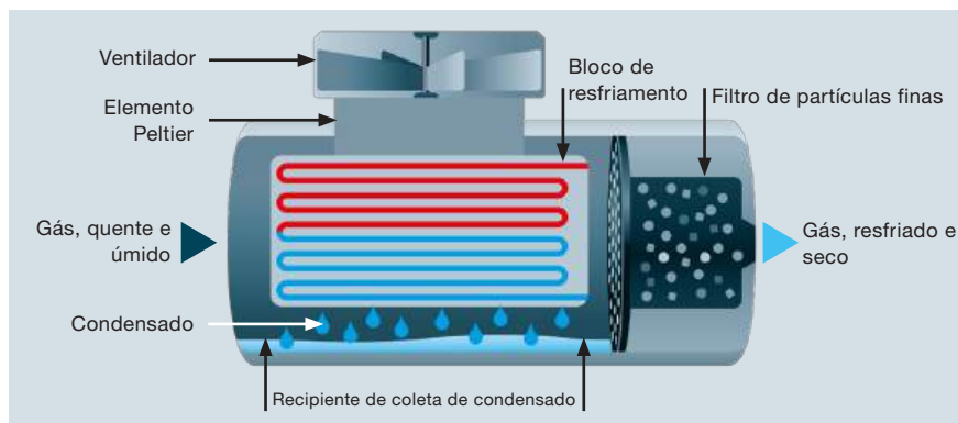
Figura 58 Esquema do condicionamento de gás da Testo
