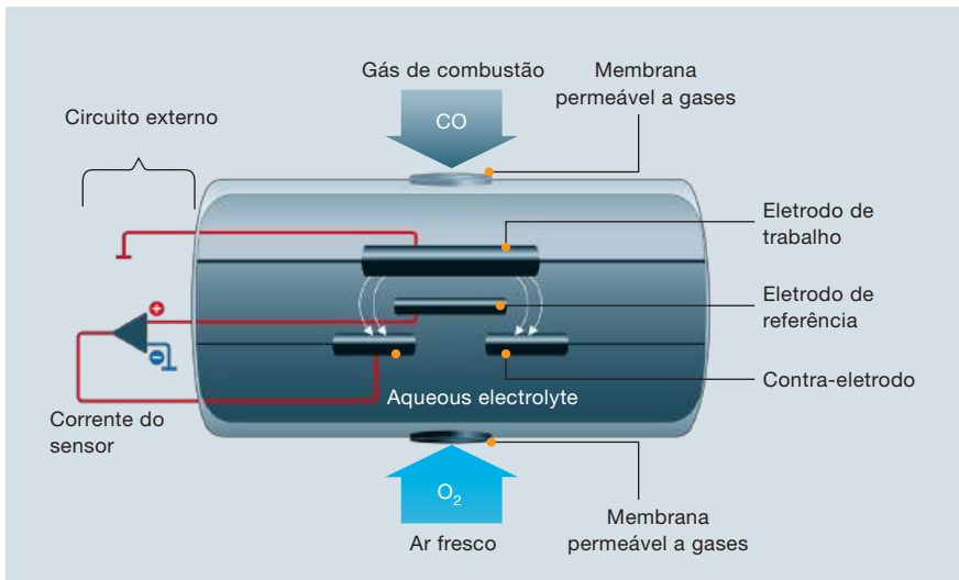
Figura 17 Sensor para CO e outros gases (esquemático)
