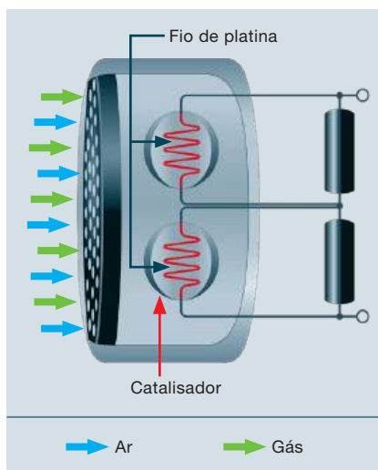
Figura 22 Sensor baseado no princípio do efeito de calor
